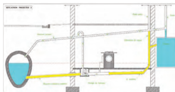
Een van de mogelijke oplossingen om via een aangepaste aansluiting de waterdichtheid tot op het straatniveau te verzekeren.
